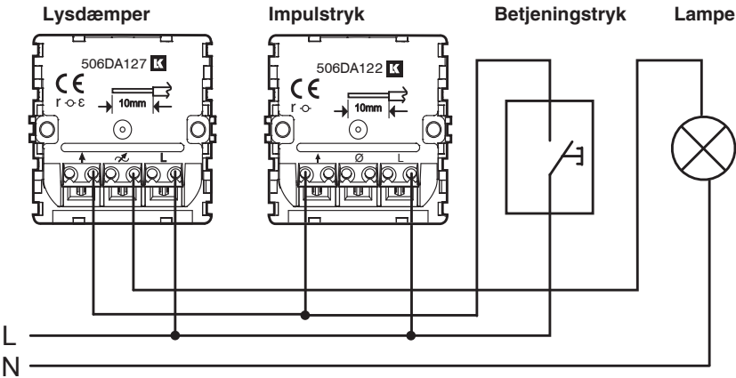
Figur 2 Lampe forbundet med lysdæmper. Her kan lysdæmperen betjenes ved tryk direkte på fronterne af lysdæmperen, impulstrykket, og på et fjederbelastet betjeningstryk.
