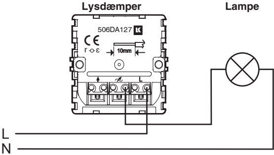
Figur 1 Lampe forbundet med lysdæmper. Lysdæmperen betjenes ved tryk direkte på fronten.
